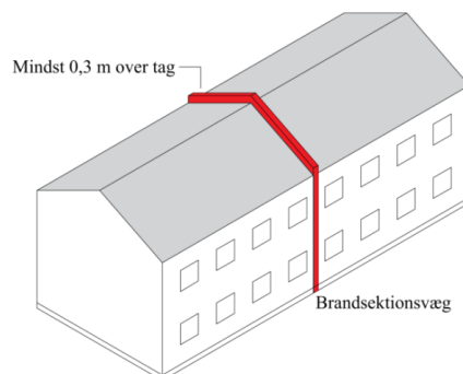
Figur 4 – Illustration af en brandkam (Figur 4.13 i BR18, Kapitel 5)
